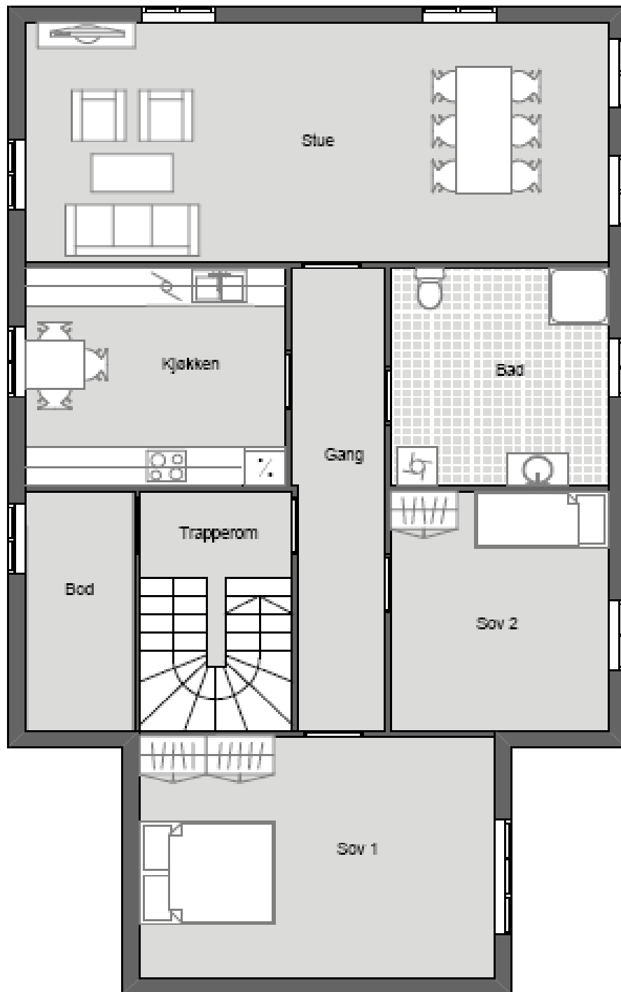
Plan 2. etasje
