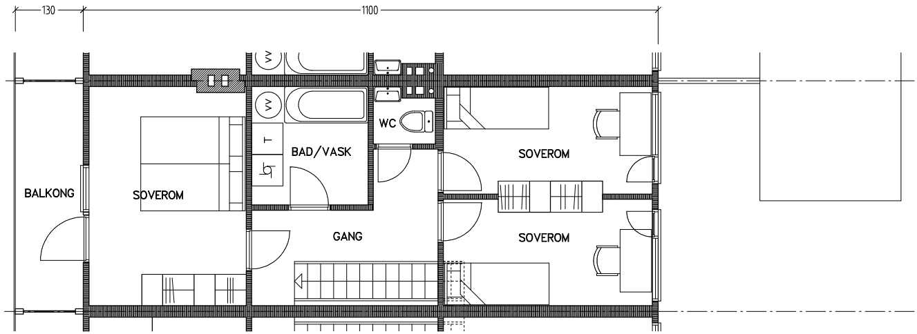
Plan 2. etasje
