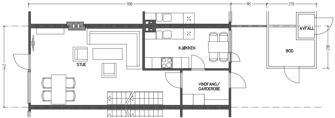
Plan 1. etasje
