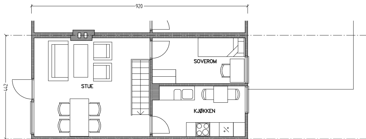
Plan 1. etasje
