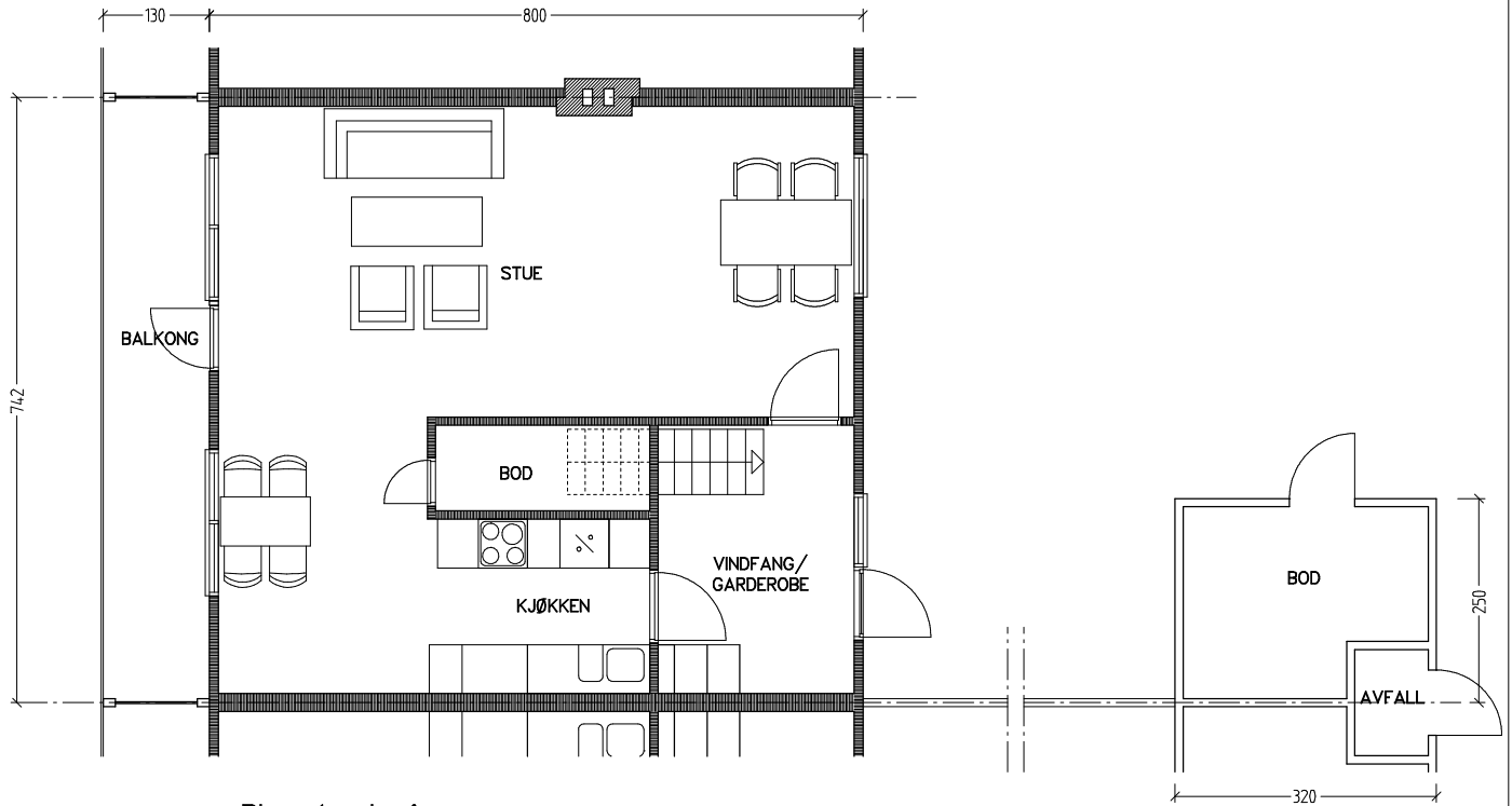
Plan 1. etasje
