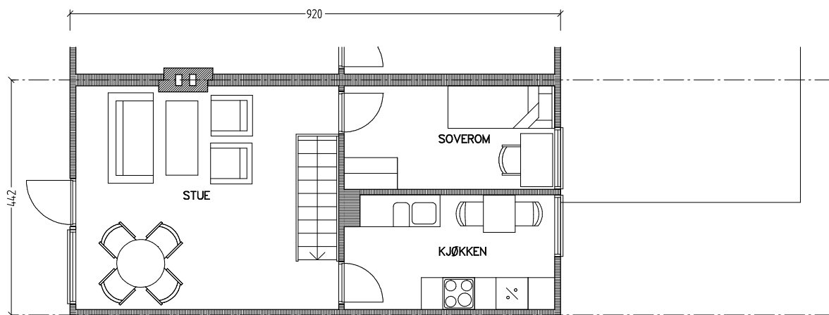
Plan 1. etasje
