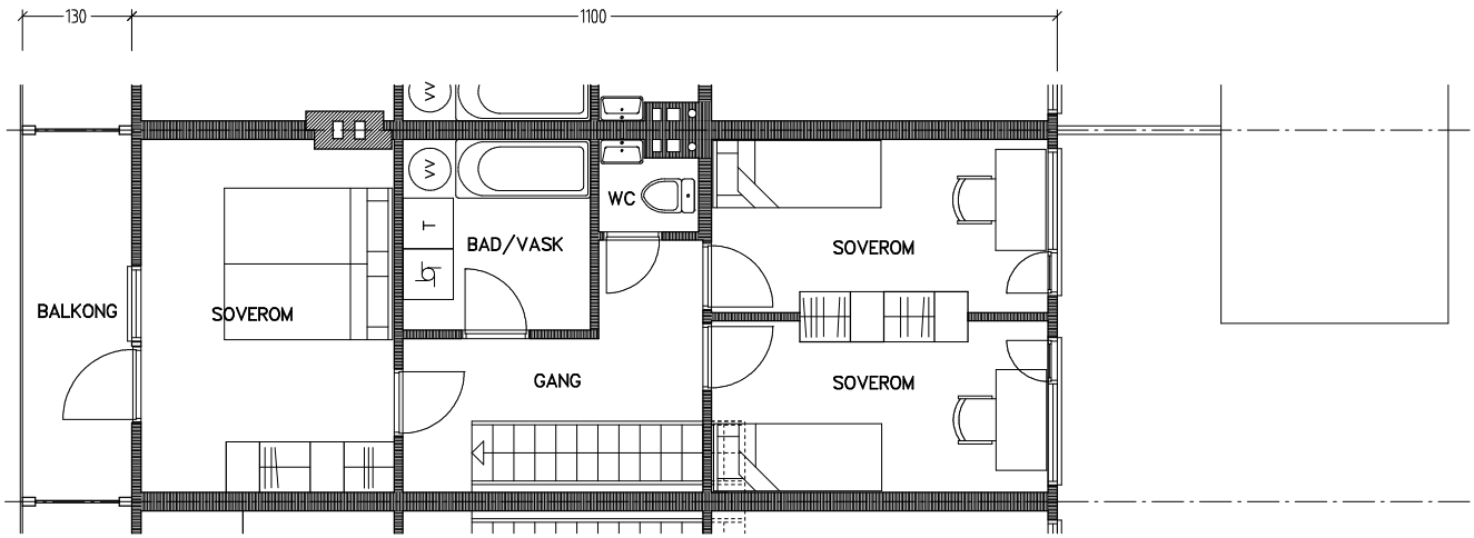
Plan 2. etasje
