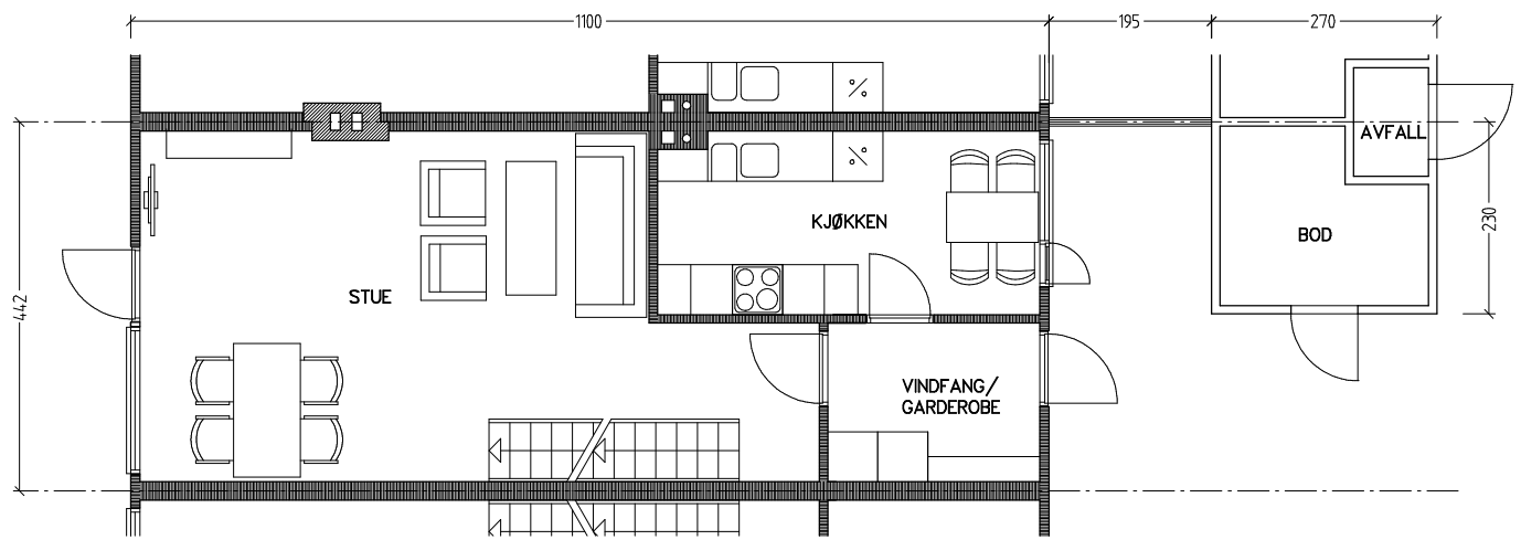
Plan 1. etasje
