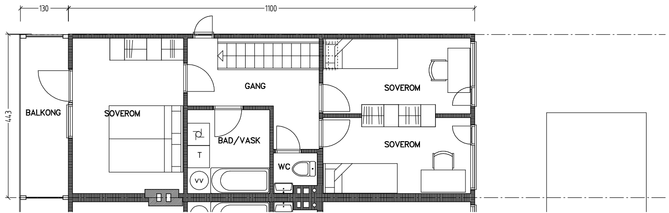
Plan 2. etasje
