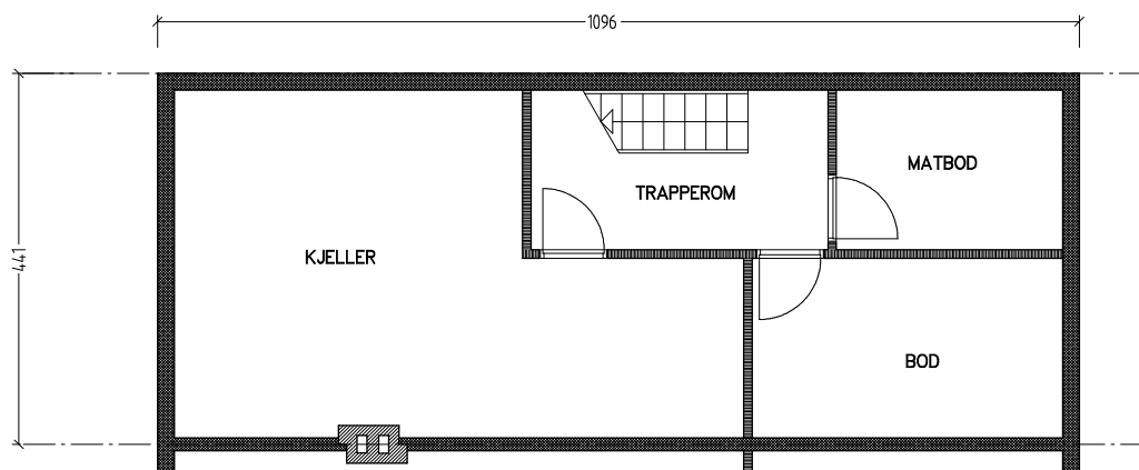
Plan kjeller
