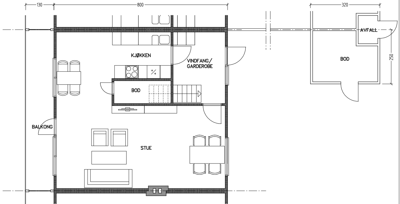
Plan 1. etasje
