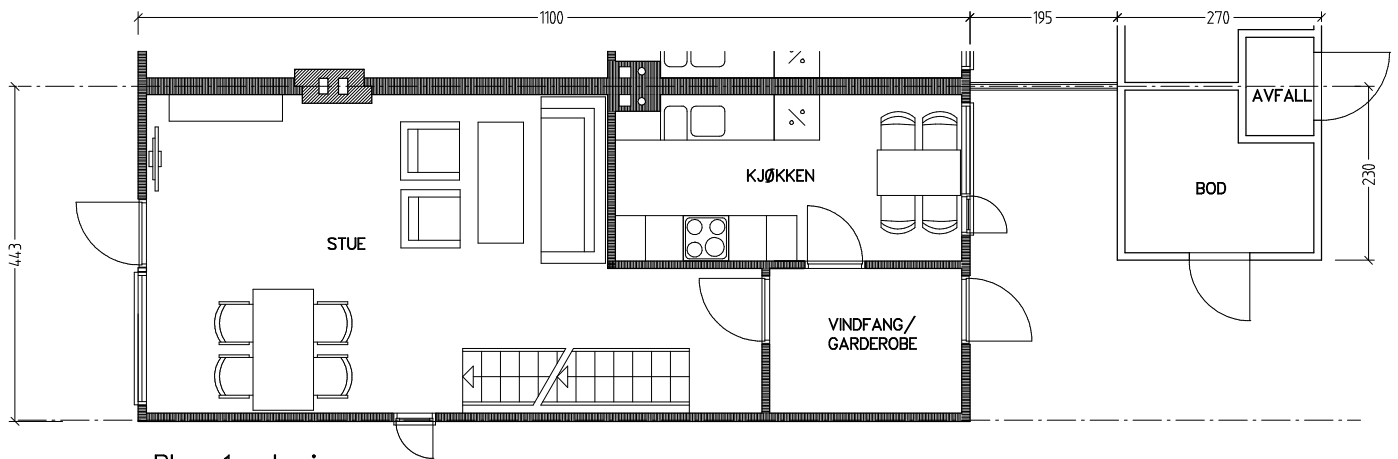
Plan 1. etasje
