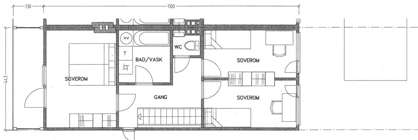
Plan 2. etasje
