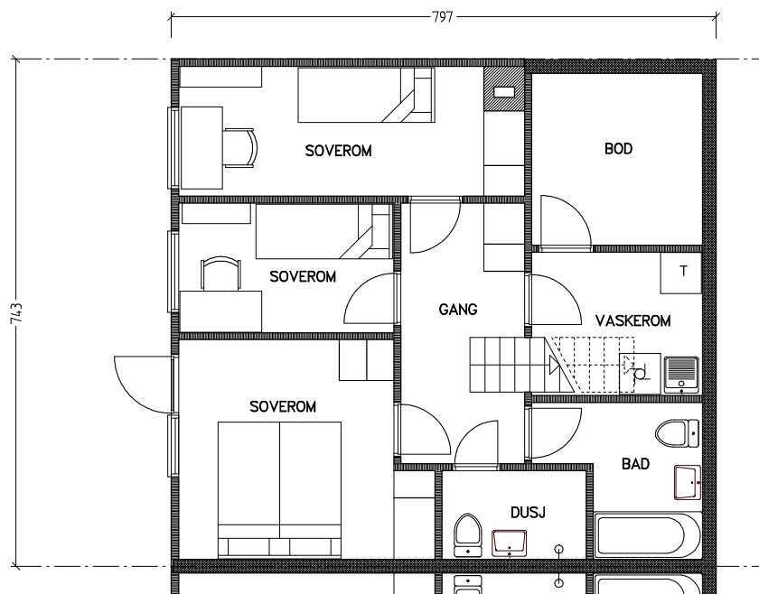
Plan u. etasje
