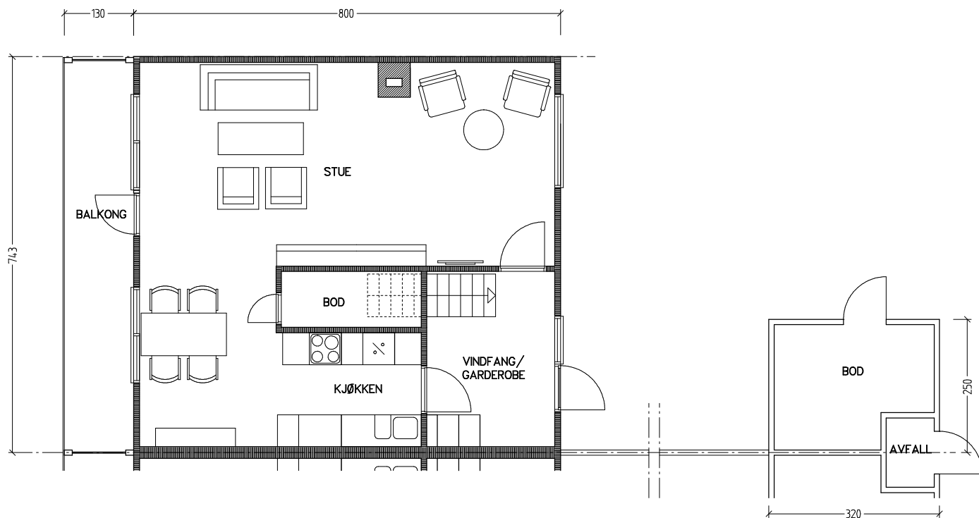
Plan 1. etasje
