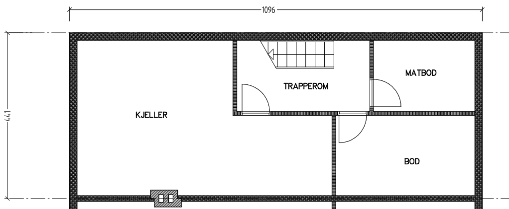
Plan kjeller
