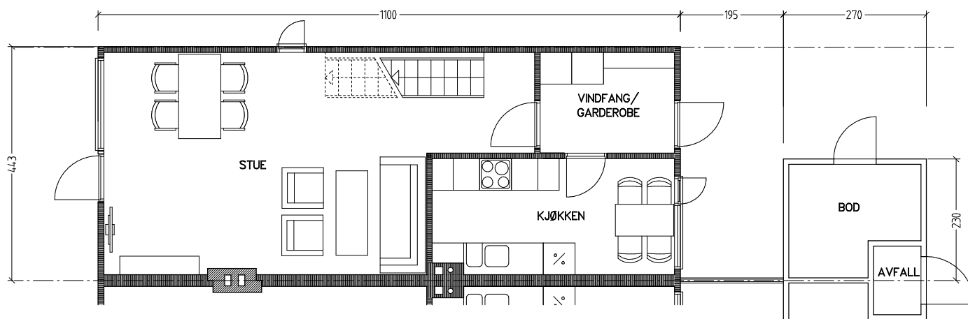
Plan 1. etasje
