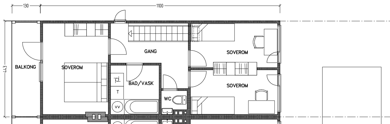
Plan 2. etasje
