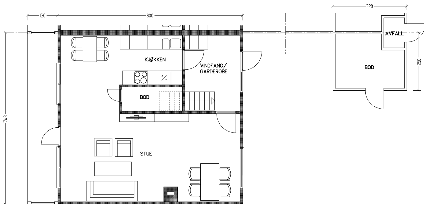
Plan 1. etasje
